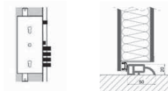
soglia con battuta singola single contact pavement threshold
